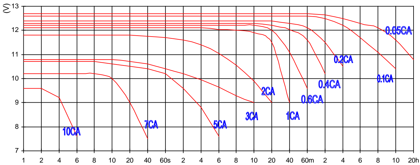
Abb.3: Entlade-Kennlinien (C=200)
