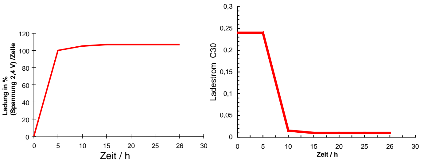
Abb.2 Zyklischer Betrieb
